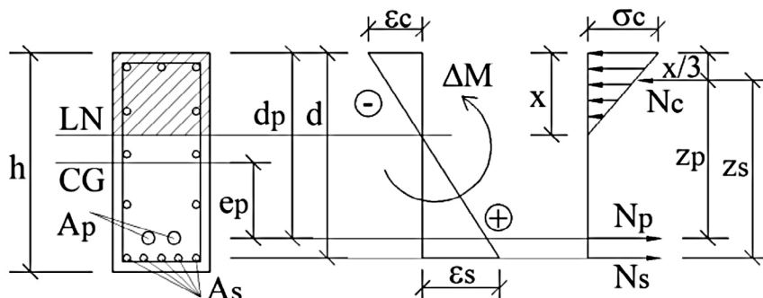
Figura 1 – Equilíbrio da seção transversal no estágio II.
