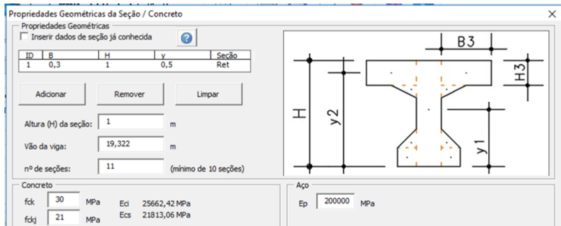
Figura 5 – Definição das propriedades geométricas da seção e materiais.
