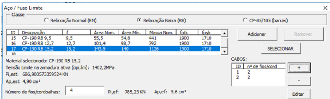
Figura 7 – Definição da armadura ativa.
