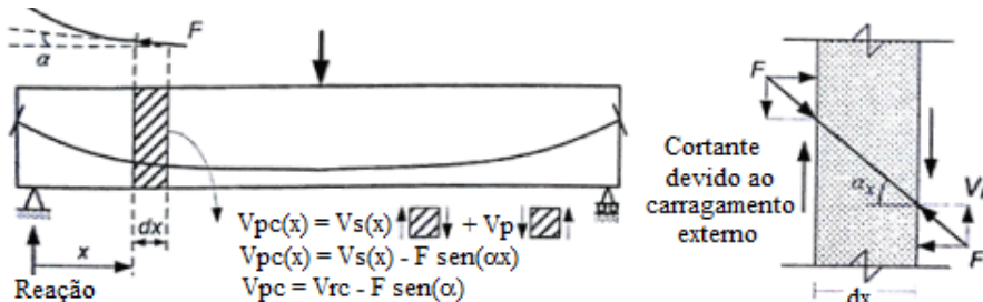
Figura 3 – Redução da força cortante no caso de cabo inclinado.
