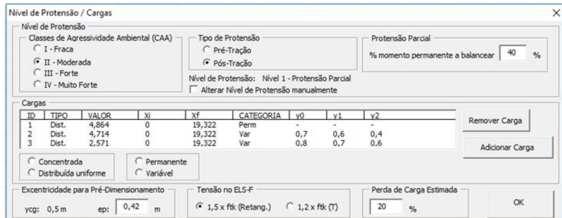
Figura 6 – Definição do nível de protensão e cargas.
