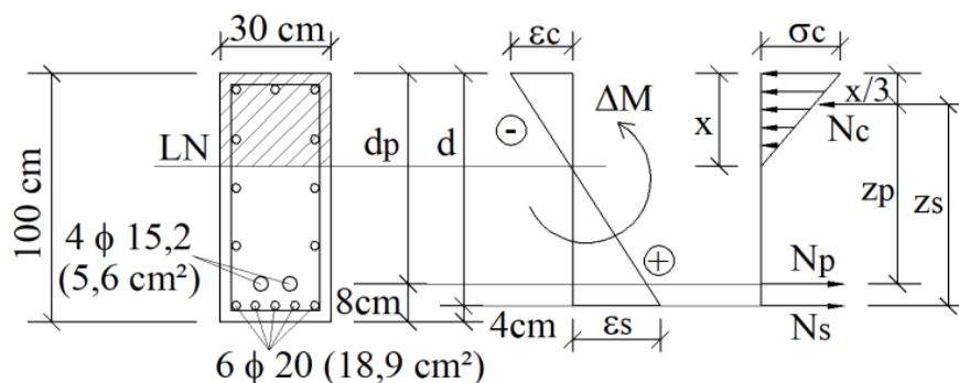
Figura 12 – Aplicação numérica: seção transversal.
