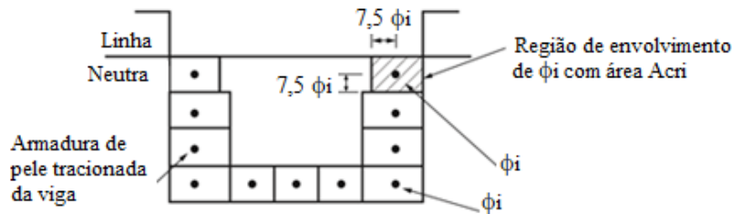
Figura 2 – Concreto de envolvimento da armadura.
