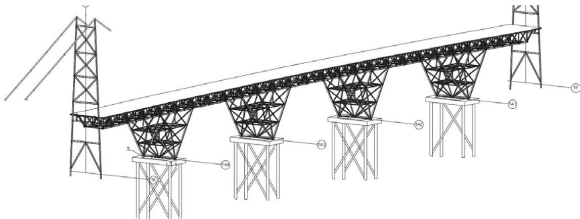
Figura 5 – Estrutura inferior auxiliar de sustentação do vão central.
