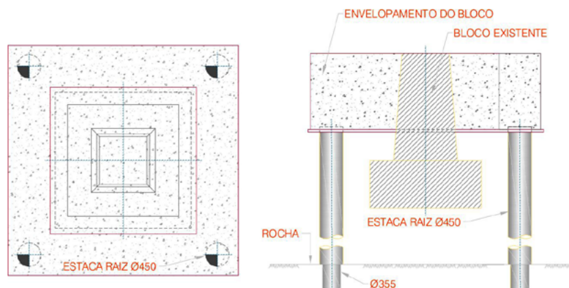
Figura 7 – Reforço típico das bases dos vãos de acesso da Ponte Hercílio Luz.
