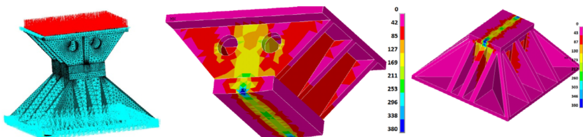
Figura 8 – Modelo e distribuição de tensões de von Mises obtidas para o apoio dos pilões [Mpa].
