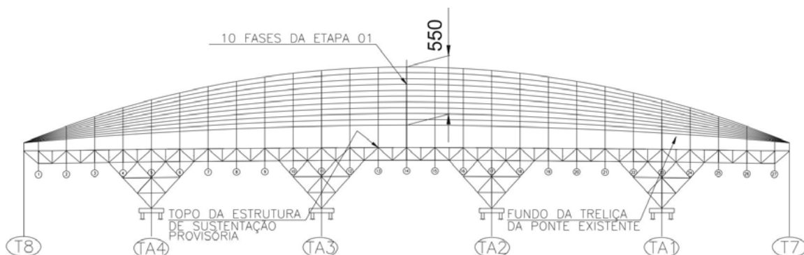
Figura 6 – Etapas da Fase 1 da transferência de cargas.
